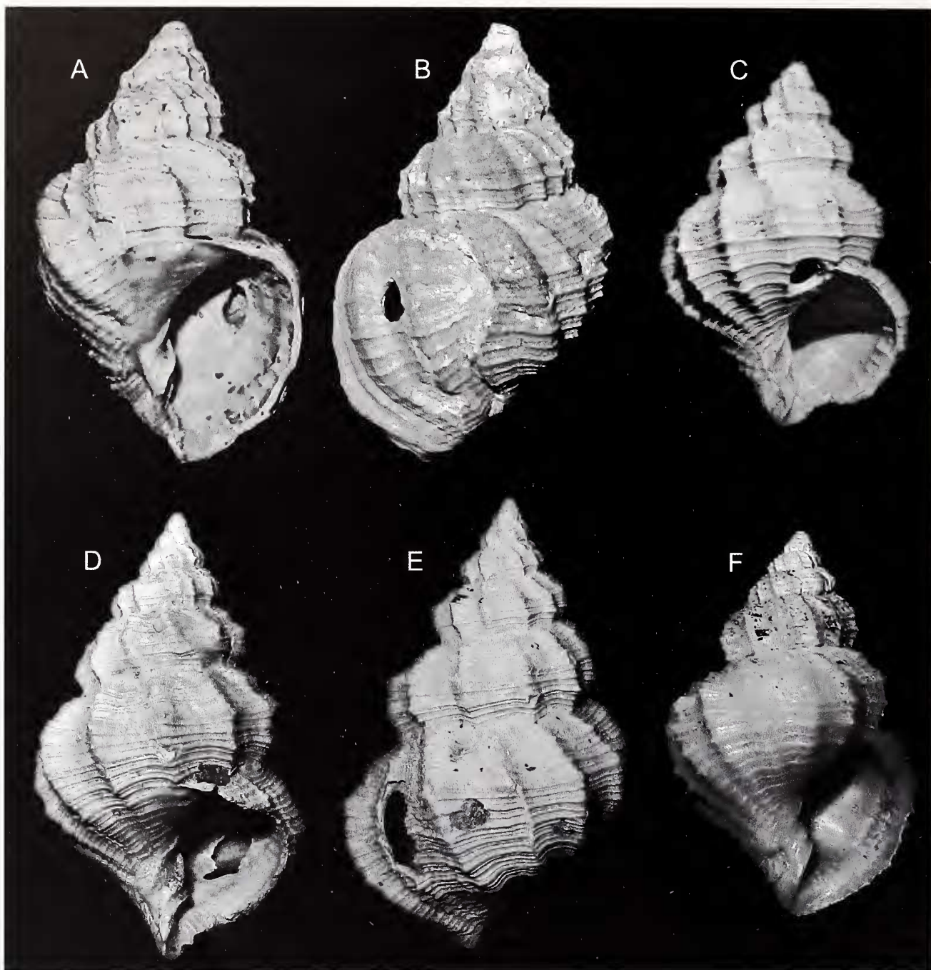
Fig. 5. Bonellitia striatissima n. sp. A, B Olotipo, Cava Campore (Parma), Piacenziano, H = 16,4 mm (MZB25718). C. Cava Campore (Parma), Piacenziano, H = 15,2 mm (ex coll. Candini MZB25721). D, E. Paratipo 1, Cava Campore (Parma), Piacenziano, H = 22 mm (MZB25718a). F. Paratipo 2, Cava Campore (Parma), Piacenziano, H = 14,7 mm (MZB25718b).
